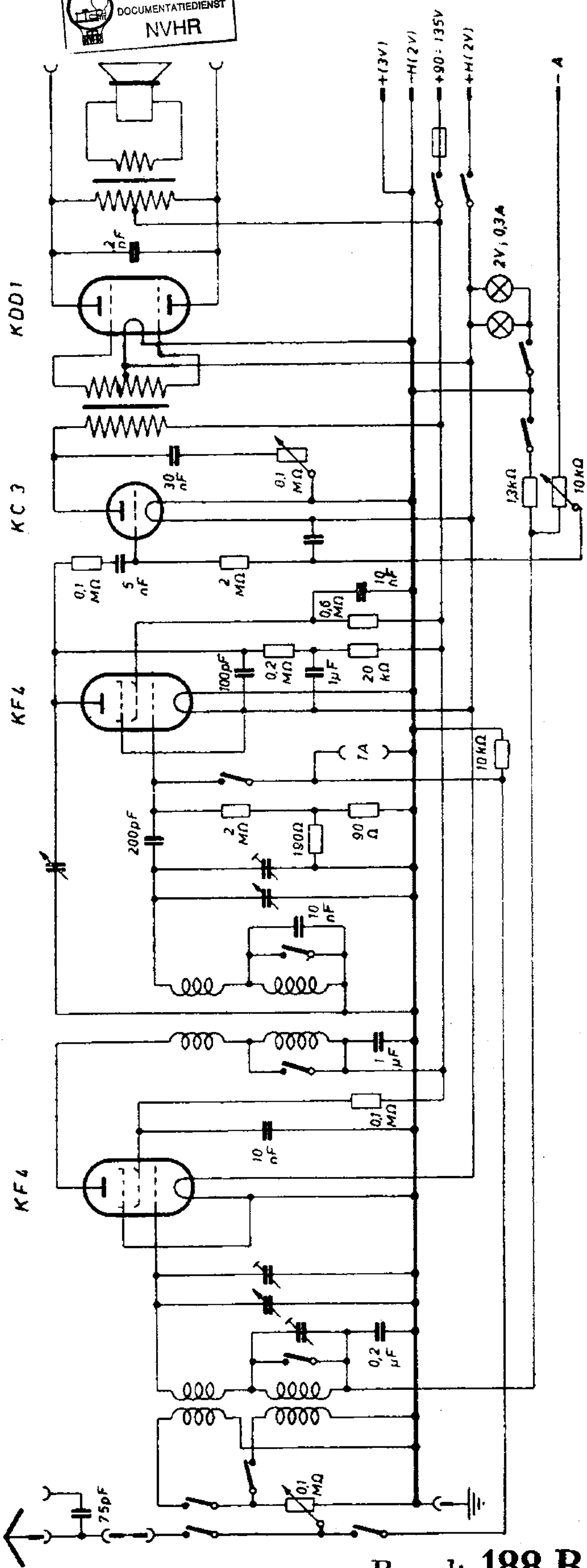
In der Rückkopplungsleitung der Audionröhre KF 4 liegt zwischen dem Drehkondensator und der Masselinie eine Spule
