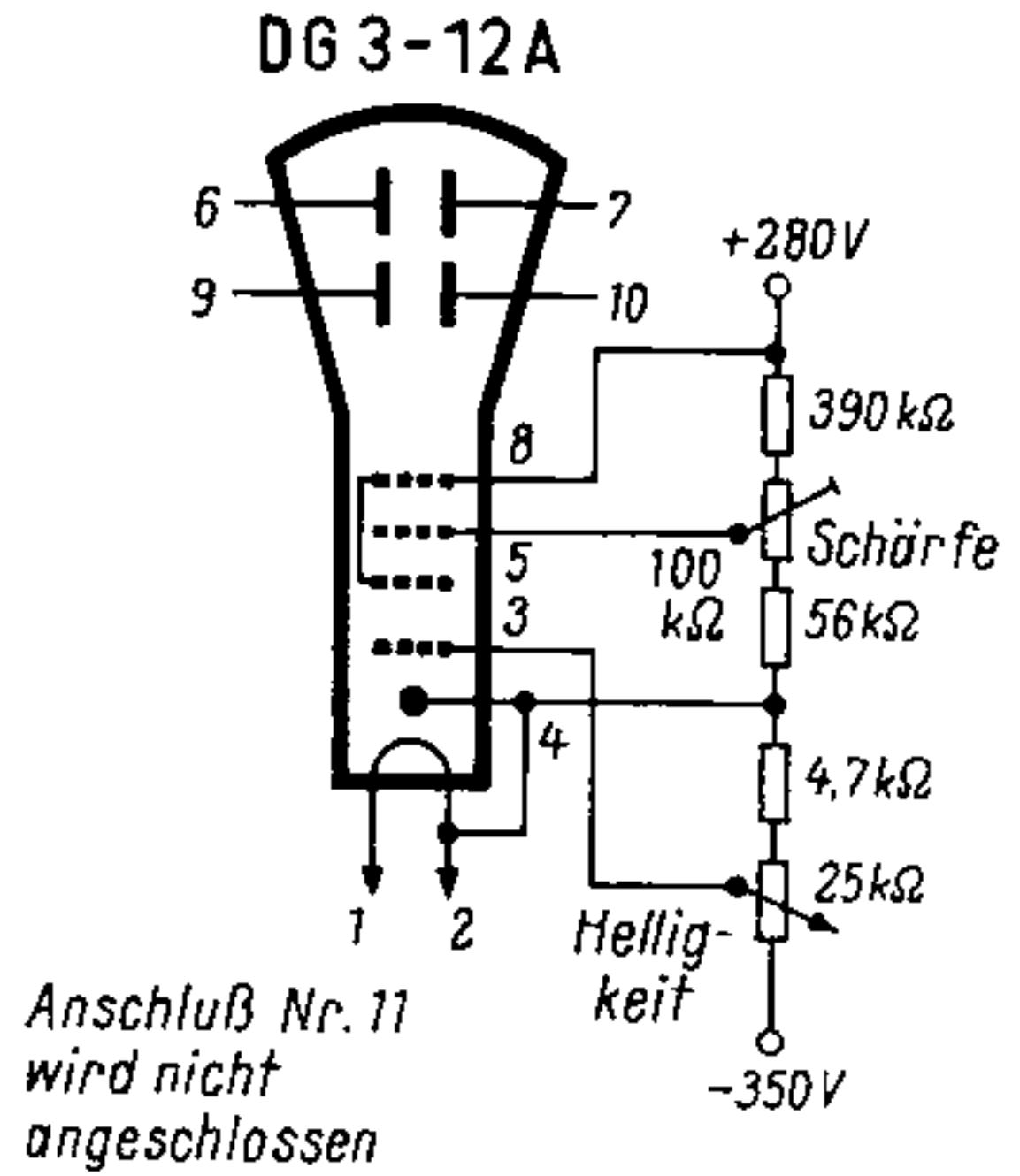
Sichtteil des Oszillografen
