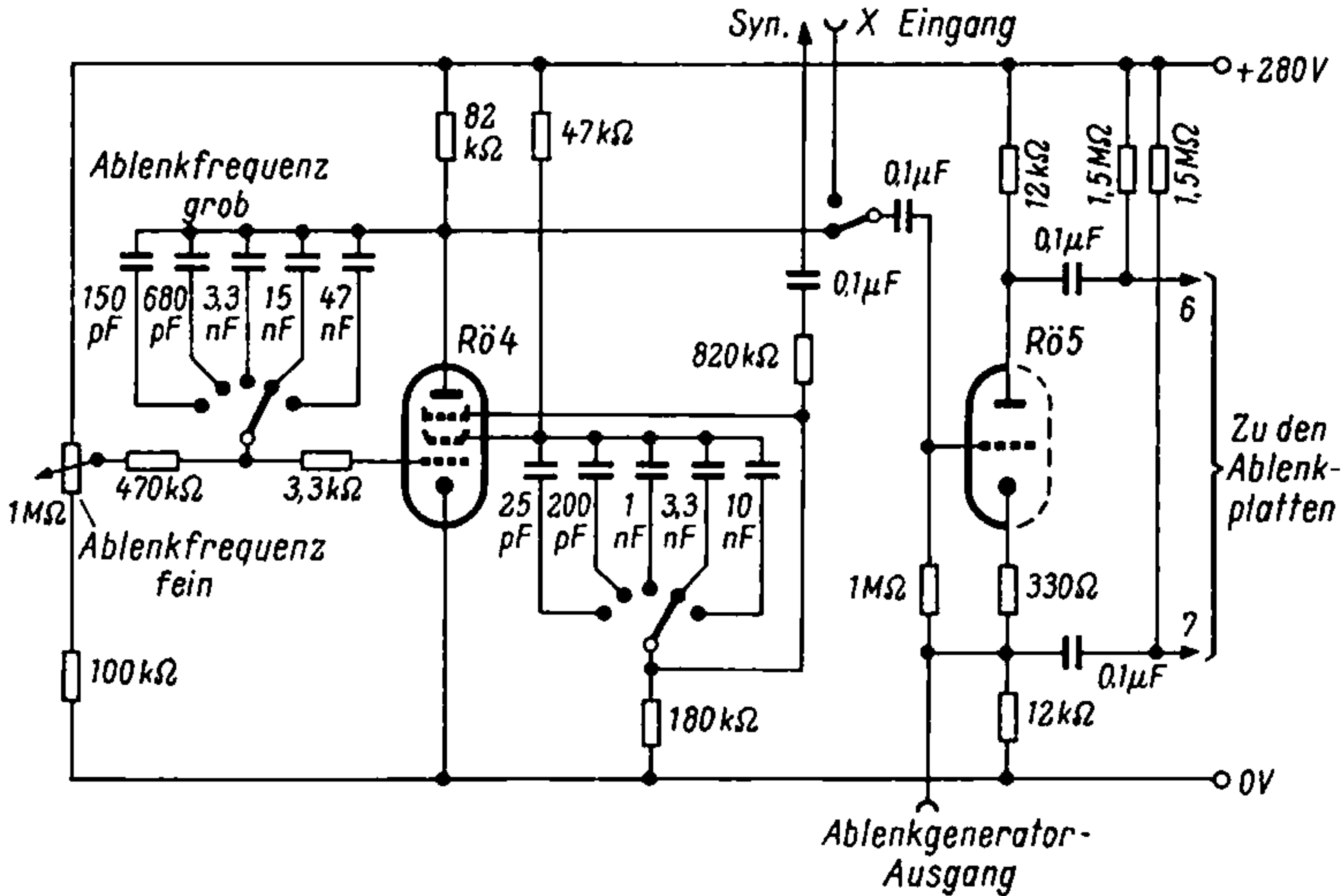
Schaltung des Ablenkgenerators. Die beiden Drehschalter sind miteinander gekoppelt
