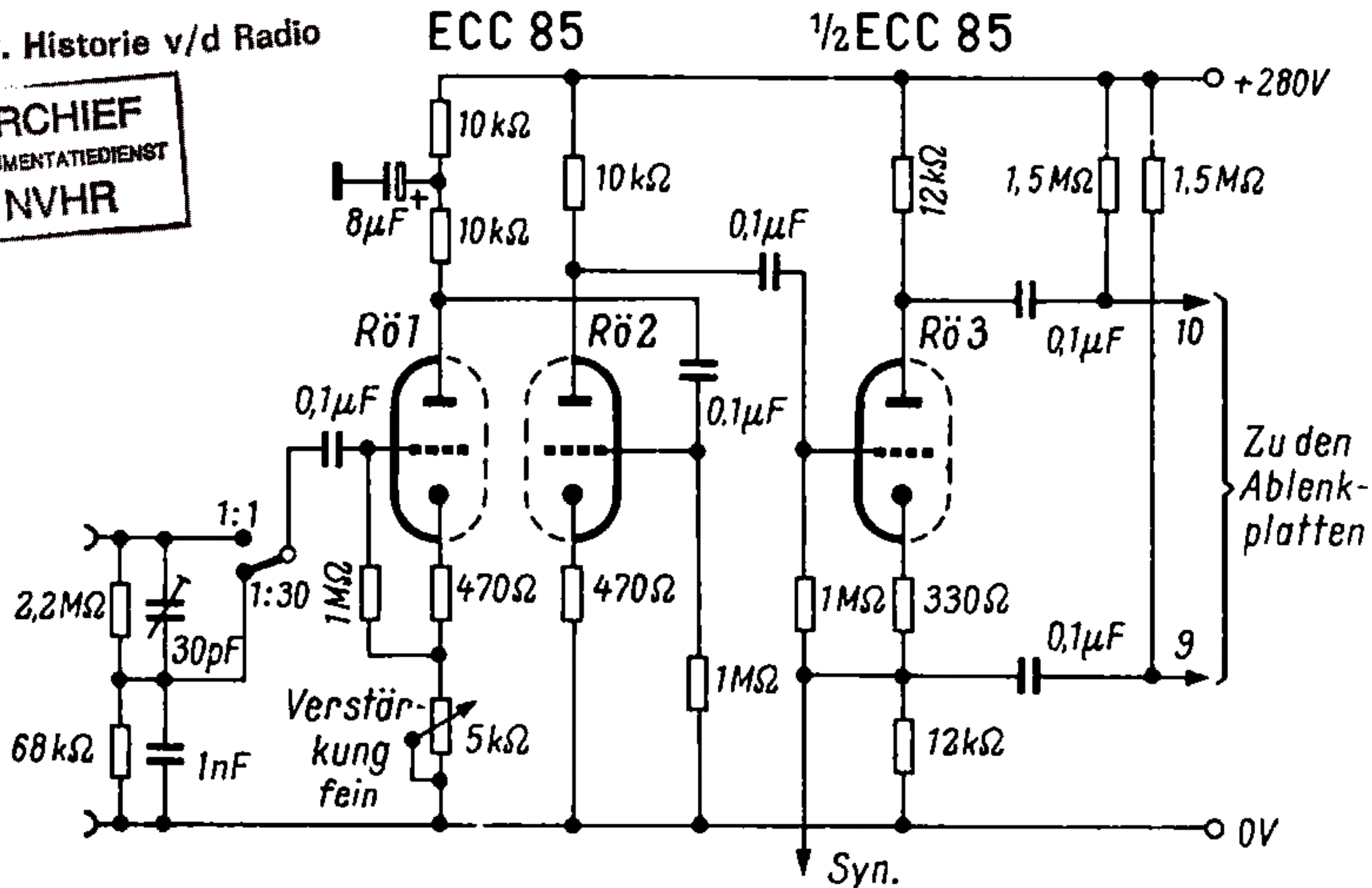
Schaltung des Y-Verstärkers. Alle Widerstände 0,5 W/10 %, sofern nicht anders angegeben
