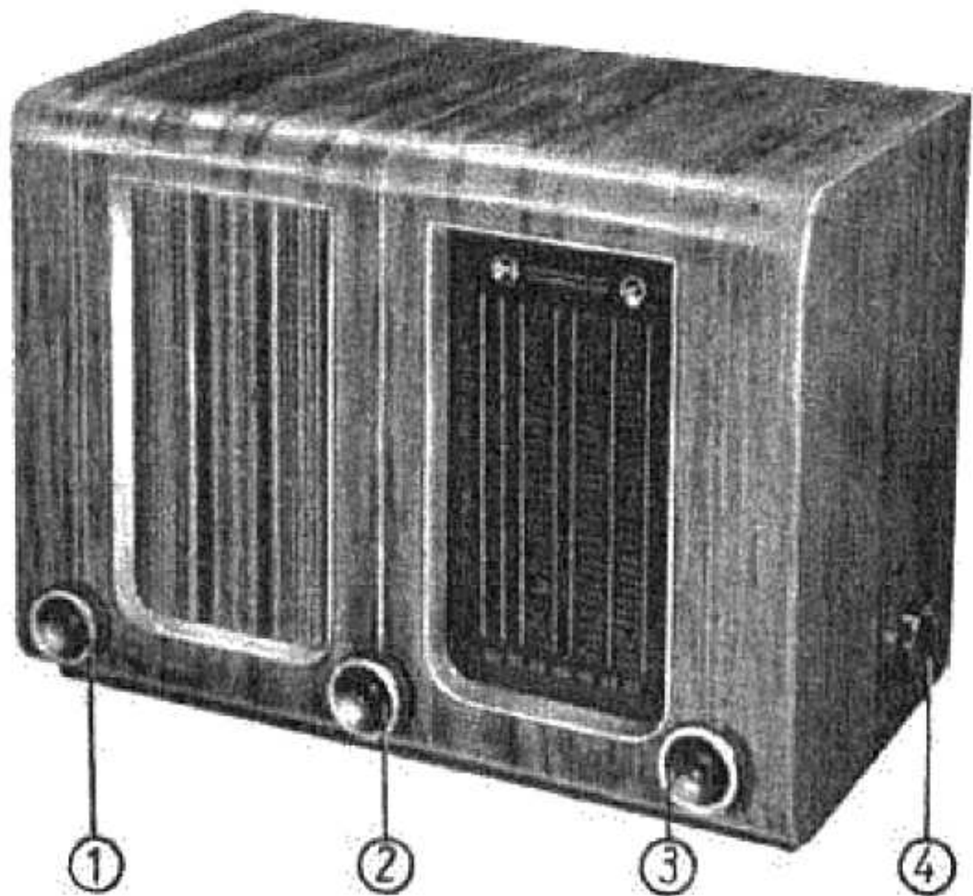
① Lautstärkereger mit Netzschalter, ② Tonblende mit Bandbreitenregelung, ③ Abstimmung, ④ Wellenbereichschalter
