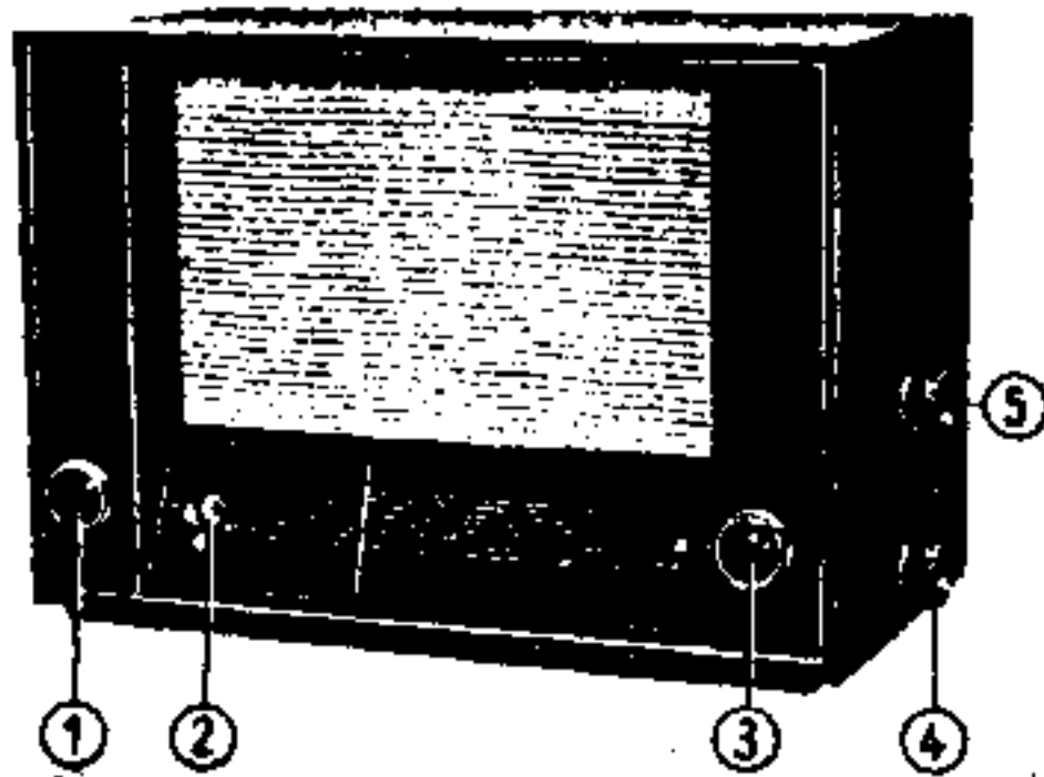
① Lautstärkereglер mit Netzschalter, ② Magisches Auge, ③ Klangblende, ④ Wellenbereichschalter, ⑤ Schwungradantrieb für Abstimmung
