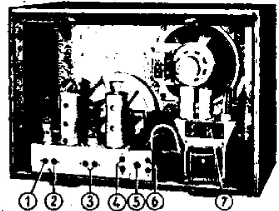
① Antennenanschluß, ② Erdanschluß, ③ Tonabnehmeranschluß, ④ Anschluß für 2. Lautsprecher, ⑤ Schalter für UKW, ⑥ Dipolanschluß, ⑦ Netzspannungswähler
