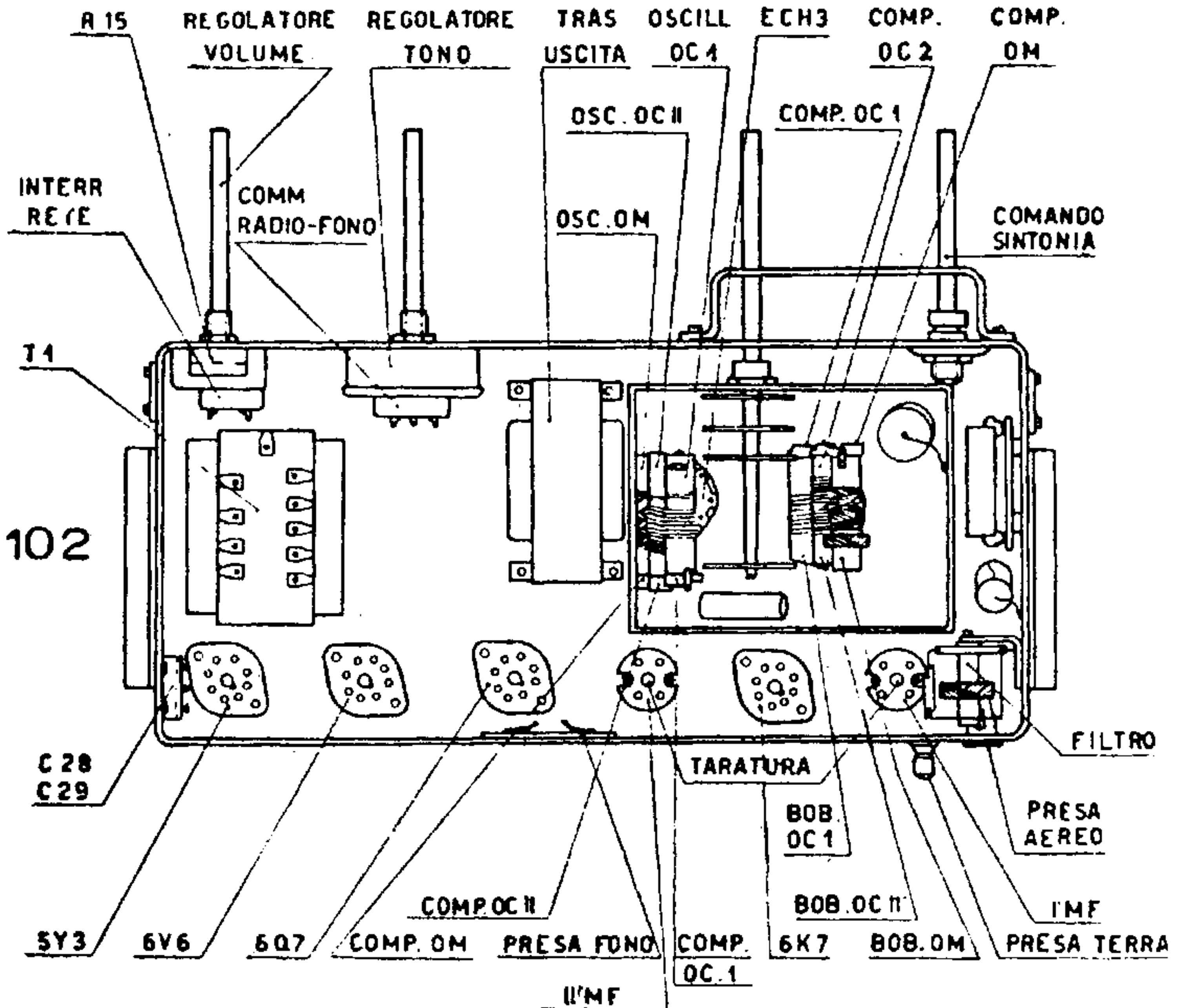
Prospetto e pianta del « 520 »
