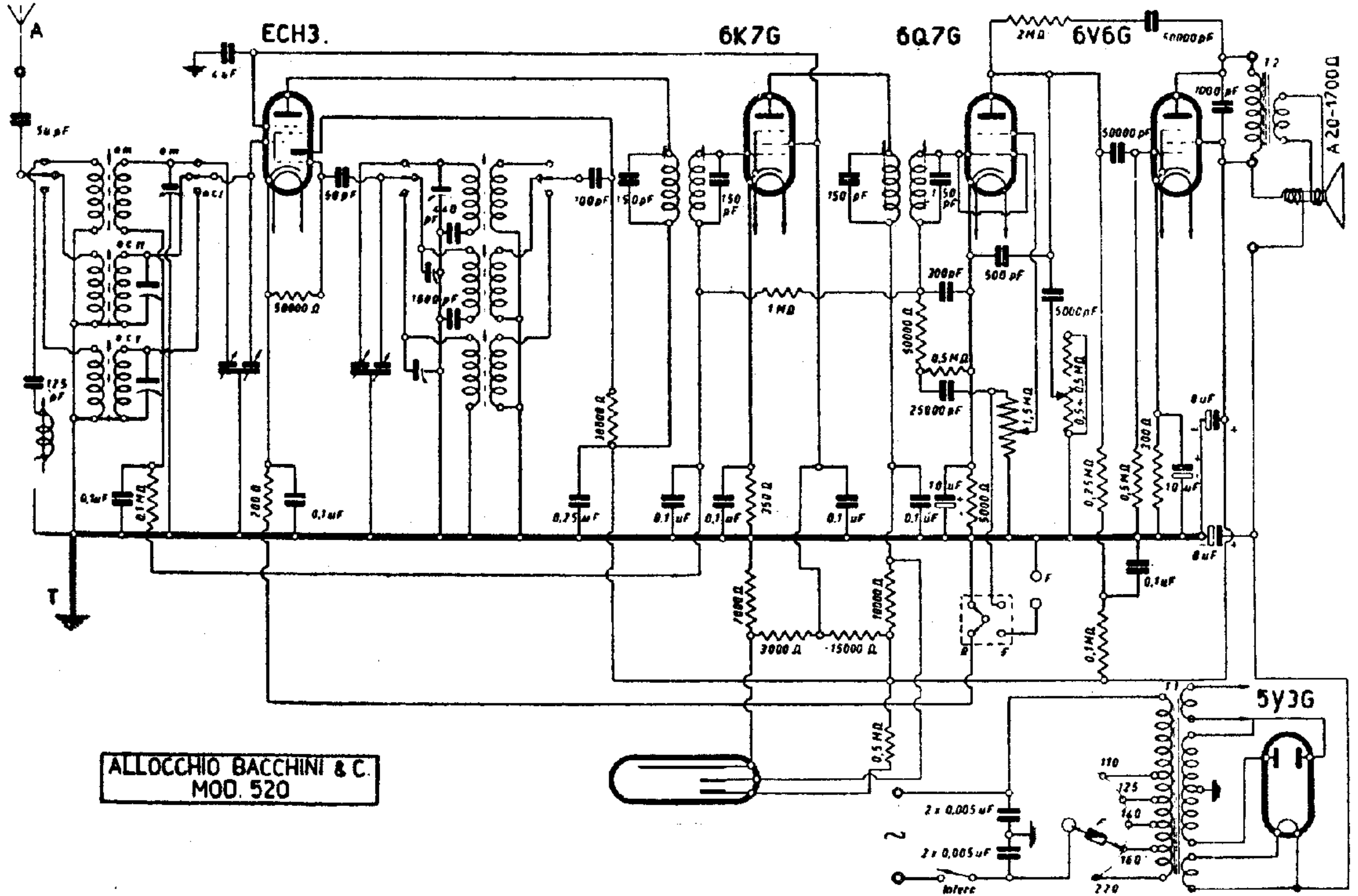
ALLOCCIO, BACCHINI & C. - MOD. « 520 »
