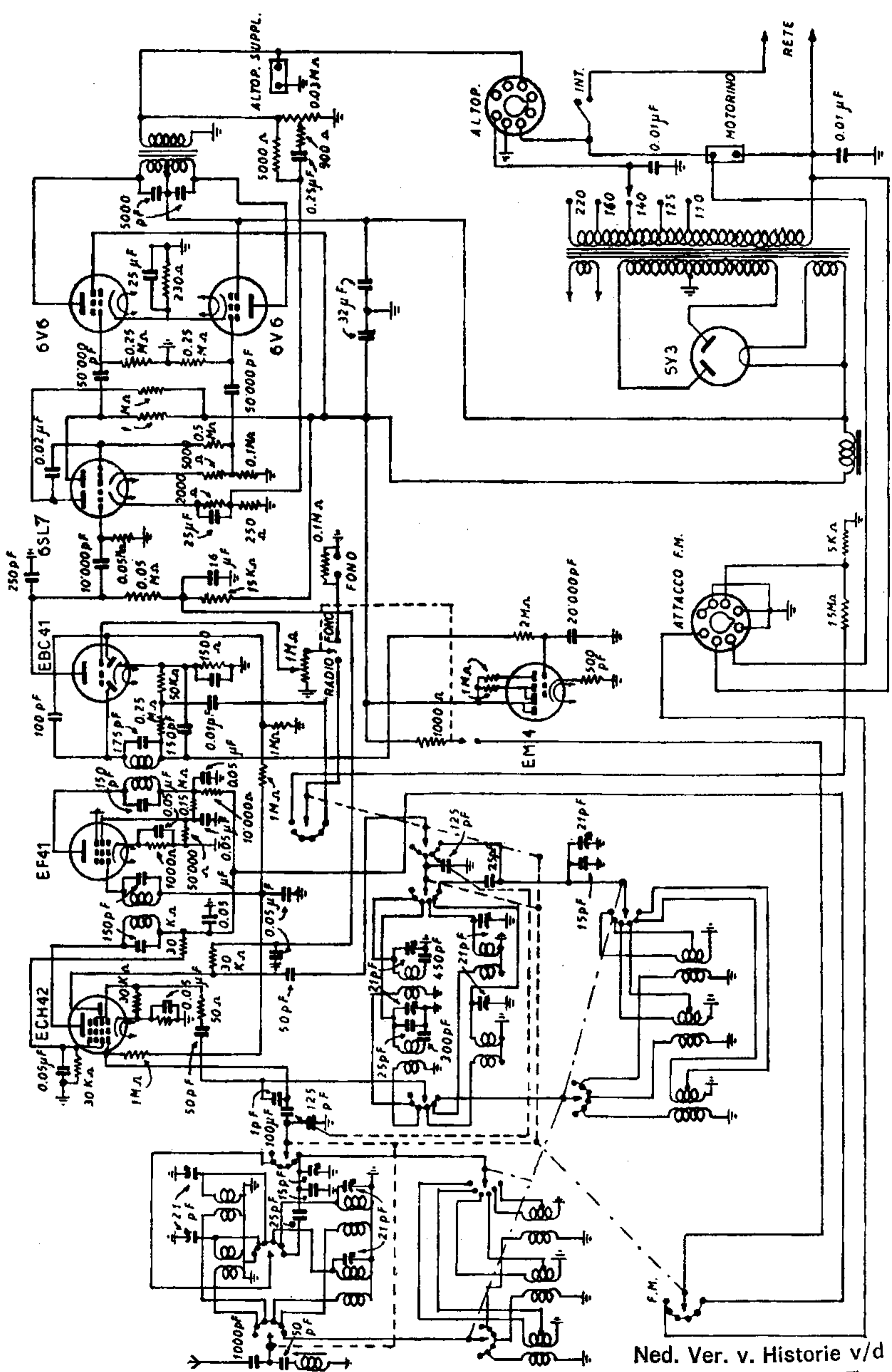
ALLOCCIO BACCHINI - Mod. 319 - Il primo triodo della SL7 amplifica il segnale a BF, l'altro triodo provvede all'inversione di fase con circuito catodina. Reazione inversa con controllo manuale. Finali in contofase classe A. Potenza d'uscita 10 watti indistoriti. Media frequenza 465 kc.
