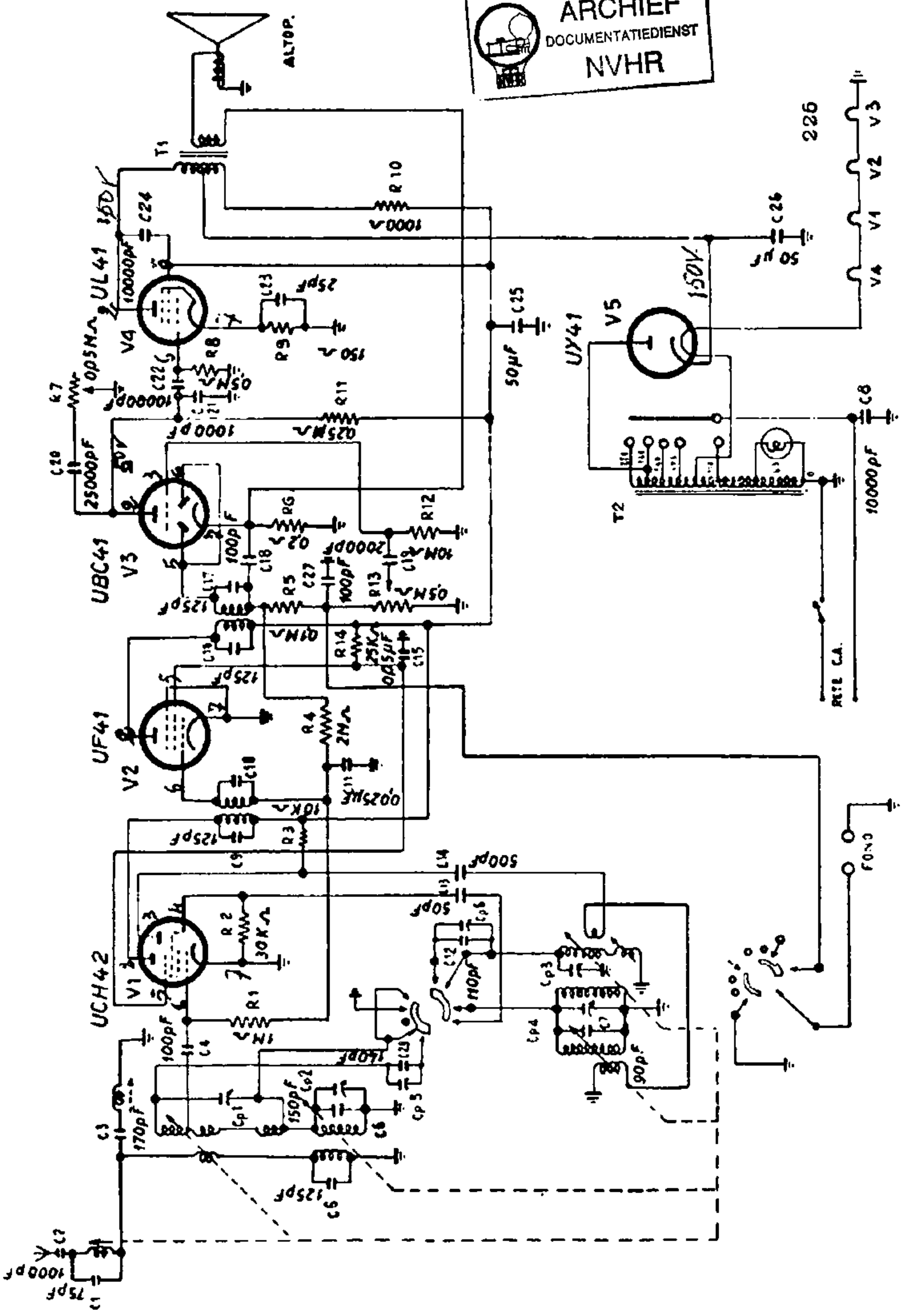
ALLOCCIO BACCHINI - Mod. 225. Ricevitore provvisto di controreazione fissa in BF. Media frequenza 465 kc.
