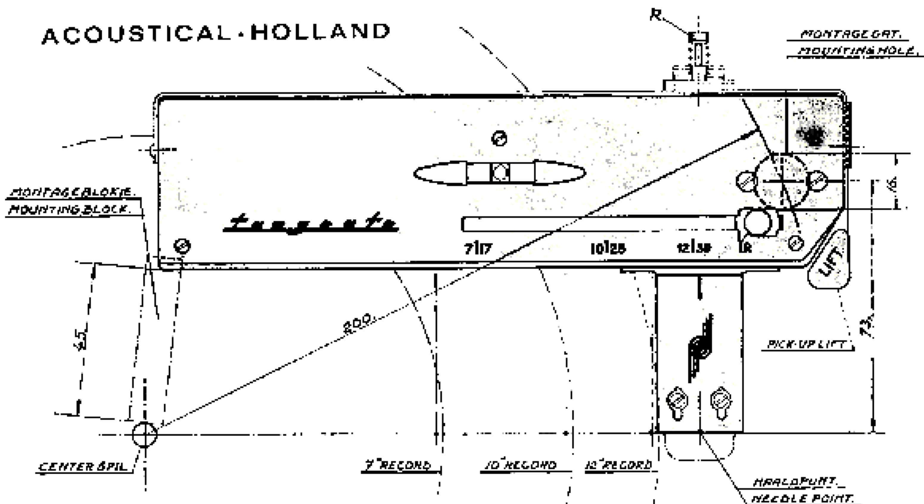
PICK-UP ARM TANGENTE BOVENAANZICHT - TOP VIEW
