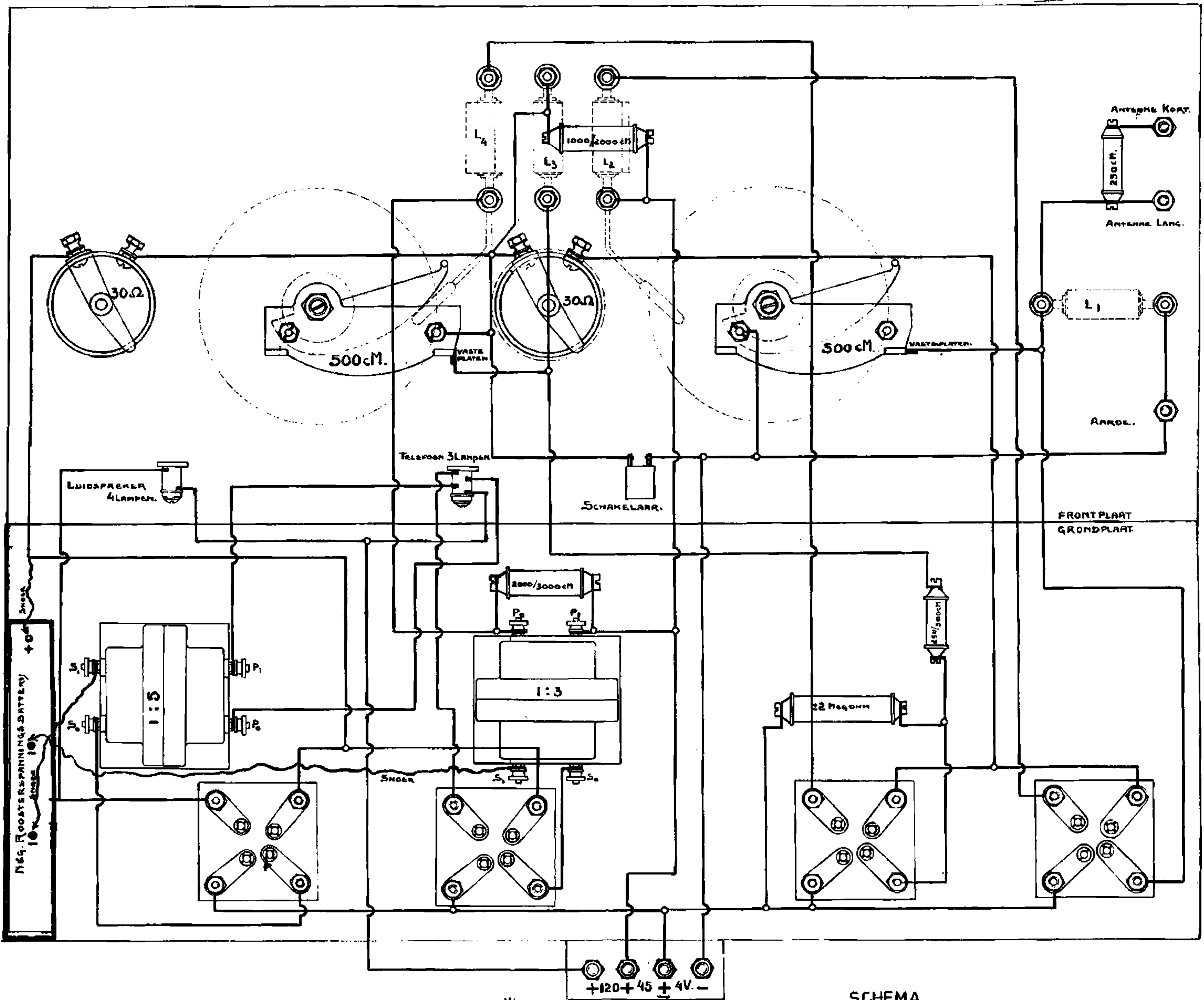
FRONTPLAAT.
