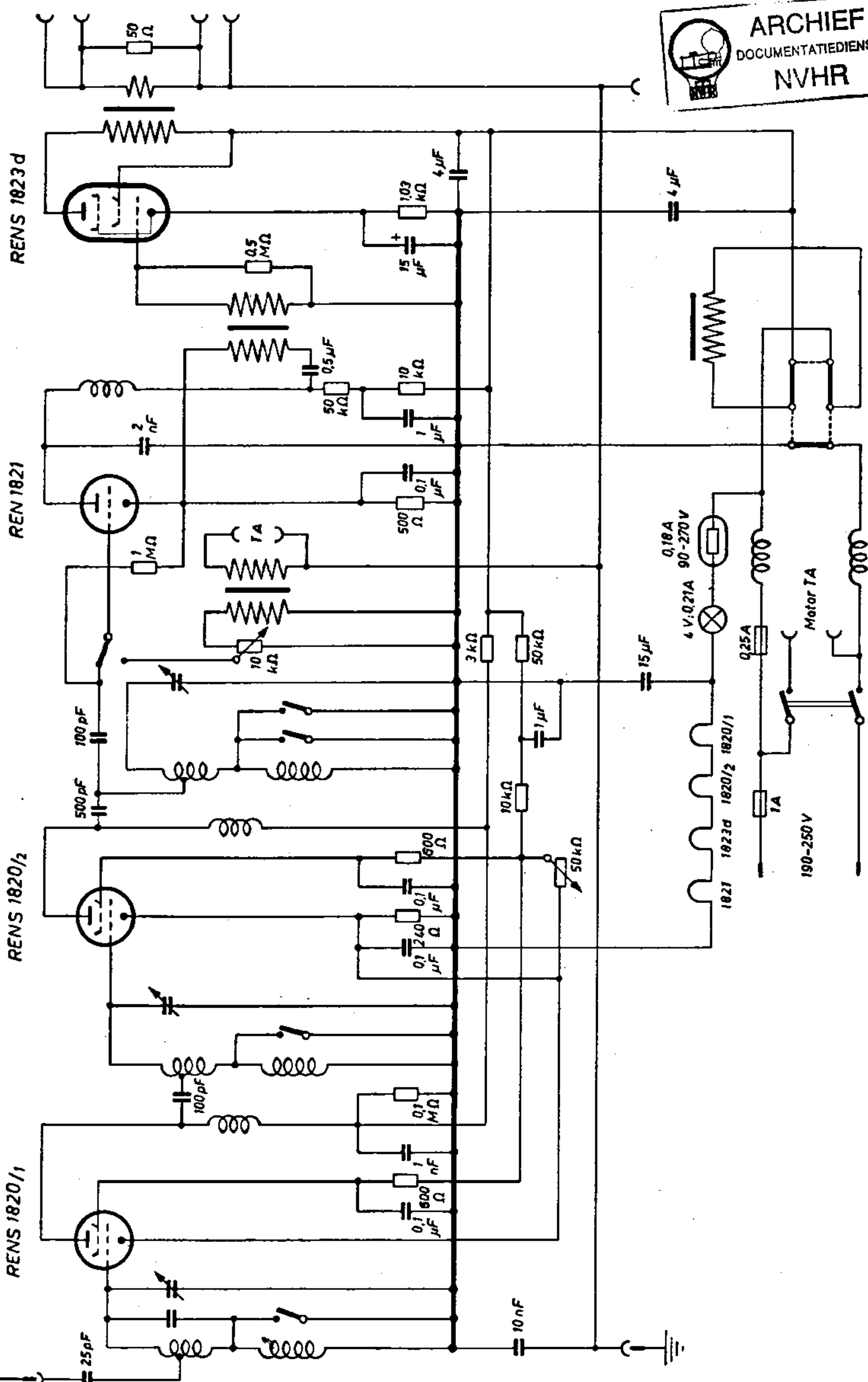
AEG Elektrola-Modell 521 G
