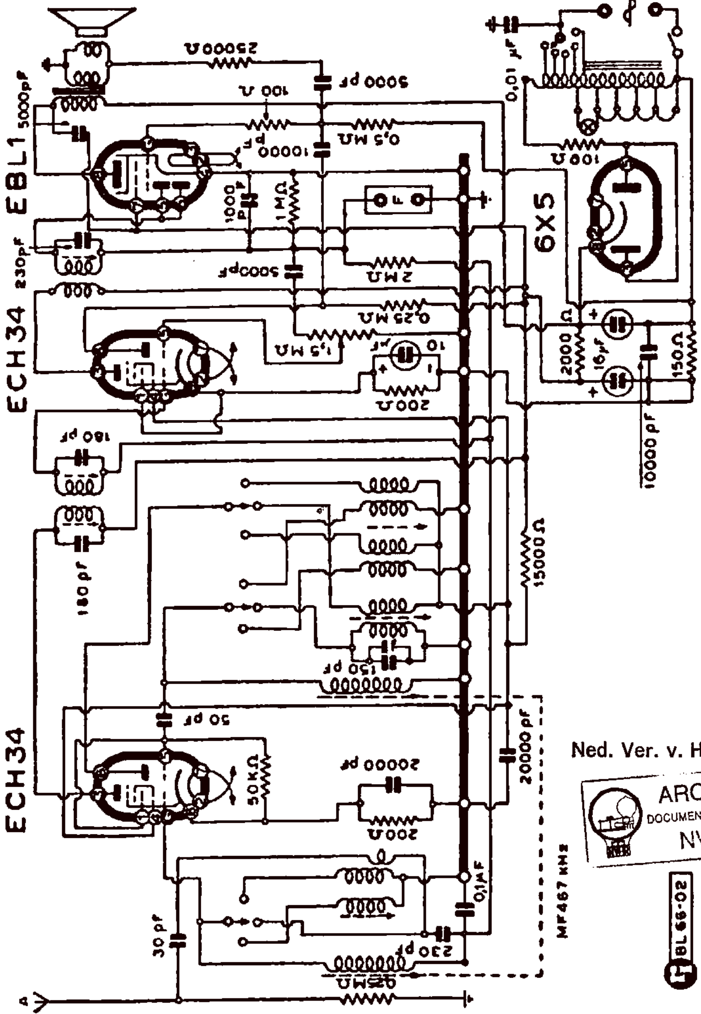
Lo schema elettrico del mod. R841
