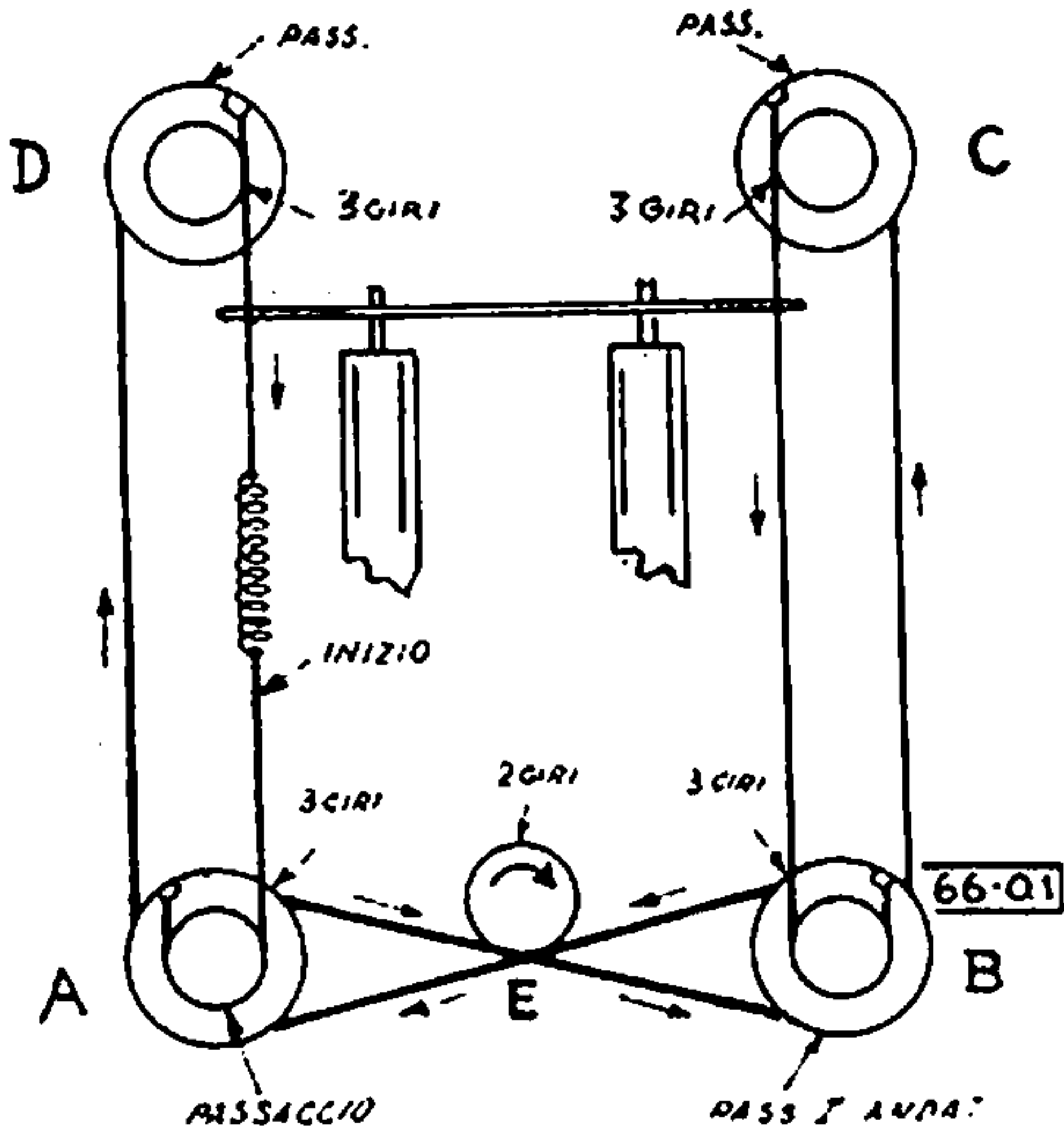
Il comando di sintonia e la funicella per l'indice del mod. « R 731 »
