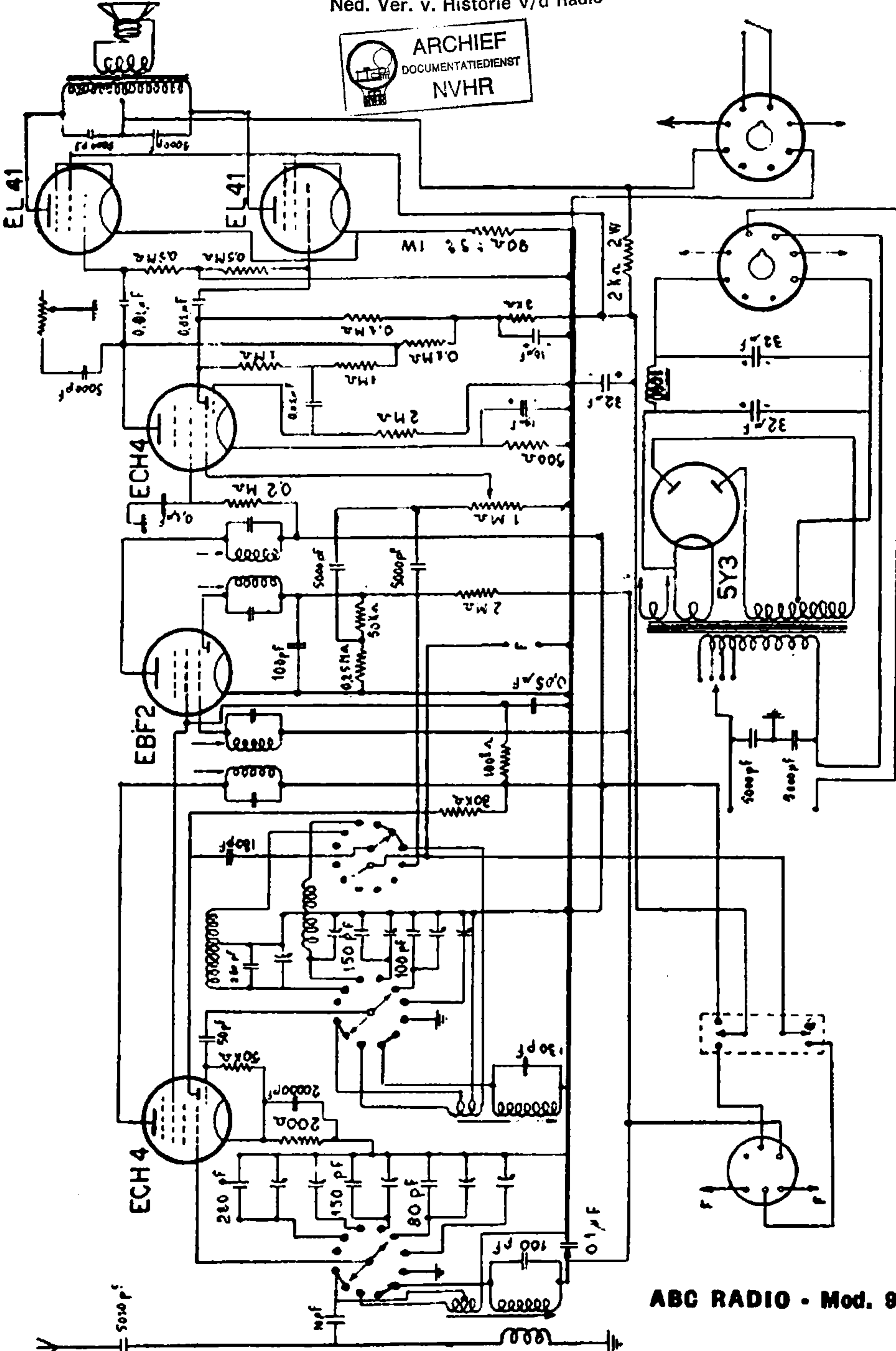
ABC RADIOCONSTRUZIONI - Mod. 972 (il mod. R 972/FM è uguale, con in più il sintonizzatore FM a cinque valvole) - Sintonia e permeabilità variabile e doppia espansione di gamma. La seconda ECH4 provvede alla preamplificazione BF e all'inversione di fase. Potenza d'uscita a 4,5 watt indistorti.
