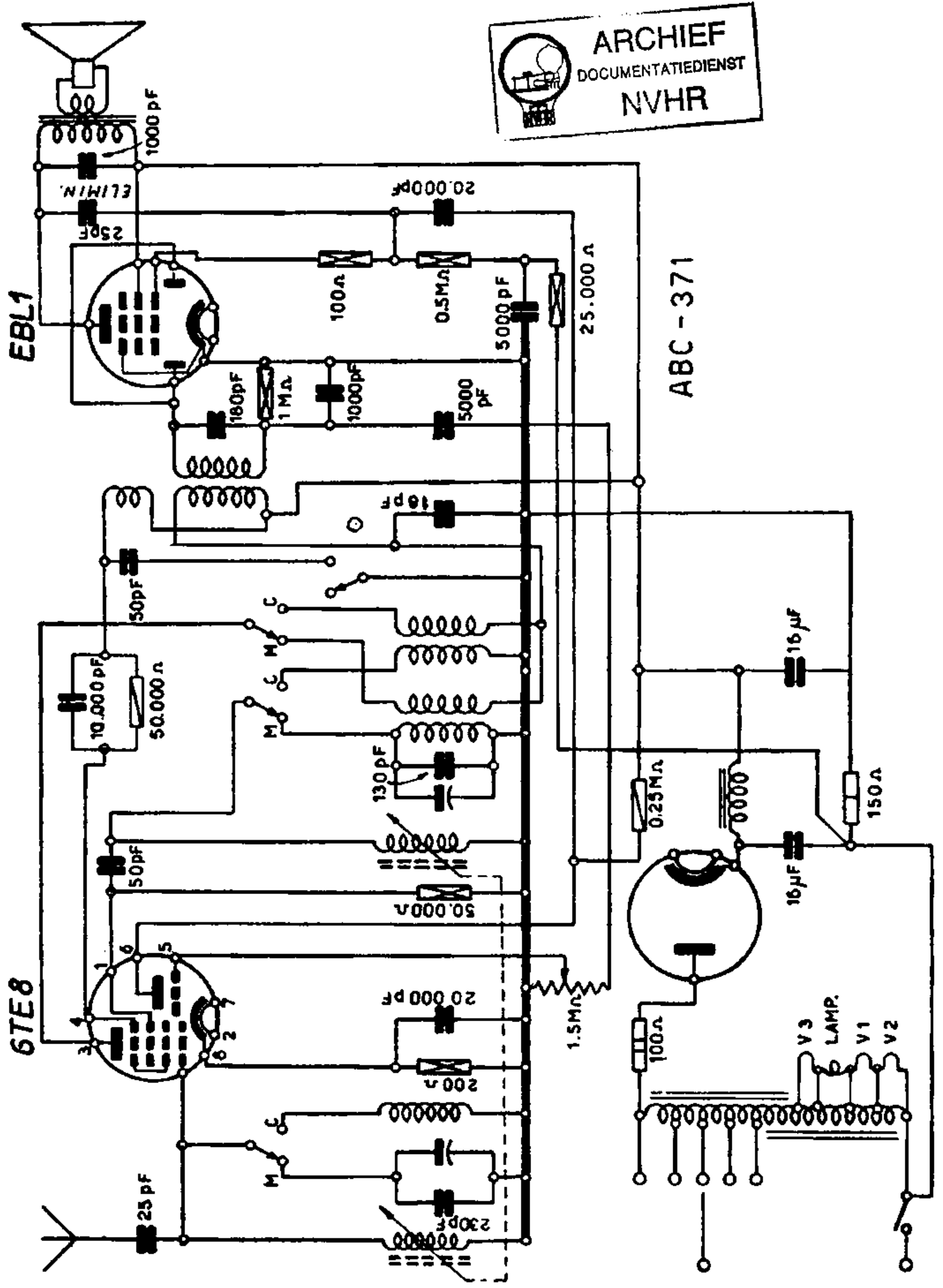
ABC RADIO - Mod. 371 - Supereterodina gamma onde medie. Valvola 6TE8 convertitrice di frequenza con exodo, e preamplificatrice BF con triodo. Valvola EBL1 rivelatrice e amplificatrice finale. Sintonia ad induttori variabili. Media frequenza 465 kc.
